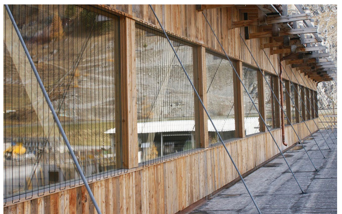
Nach wiederholtem Vogelanzprall an den spiegelnden Fenstern einer Werkhalle in S-charnf wurden nachträglich im Abstand von 8–10 cm schwarze Nylo-schnüre gespannt. Im Anschluss an die Nachrüstung wurden keine Vogelkollisionen mehr dokumentiert.
